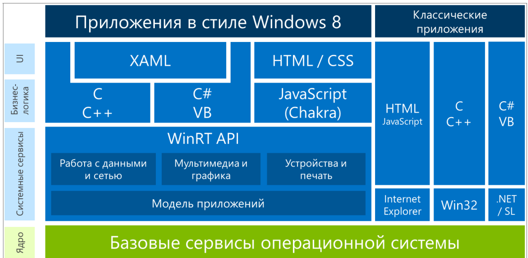
Рис. 1.7. Платформа Windows 8
