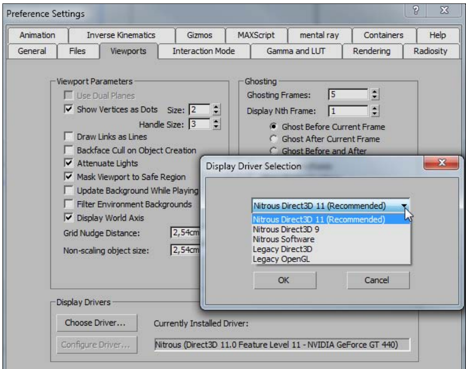
Рис. 1.13. Настройка драйверов
