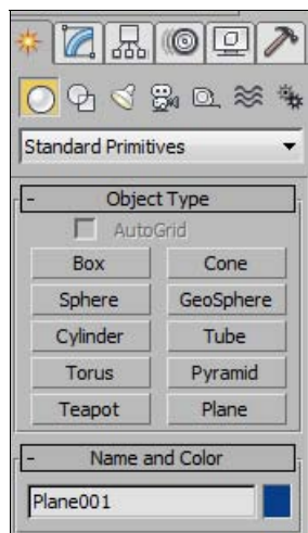
Рис. 1.4. Командная панель
